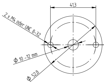
Abb. 1: Schlüssellochrosette 2226 (Türaußenseite)
